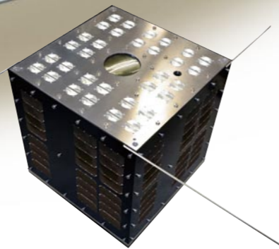
信州製可視光通信実験衛星 ぎんれい
